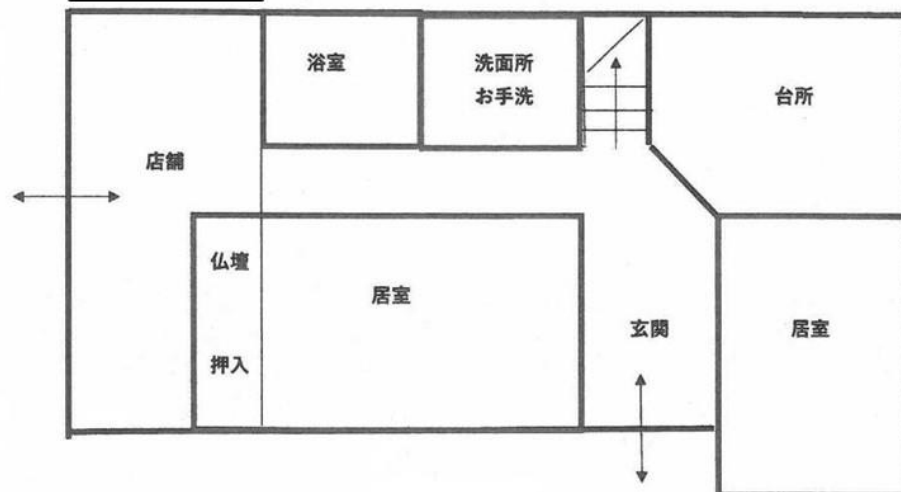
一階平面図
