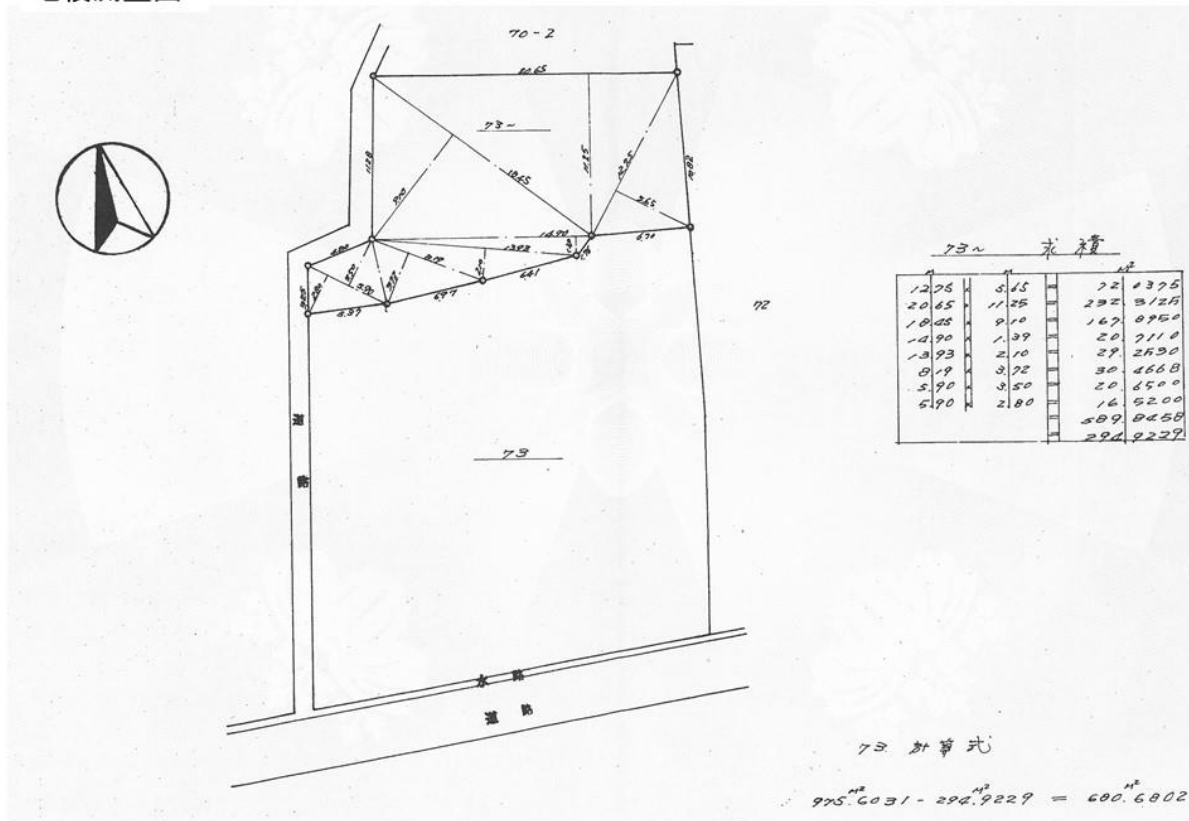
地積測量図
