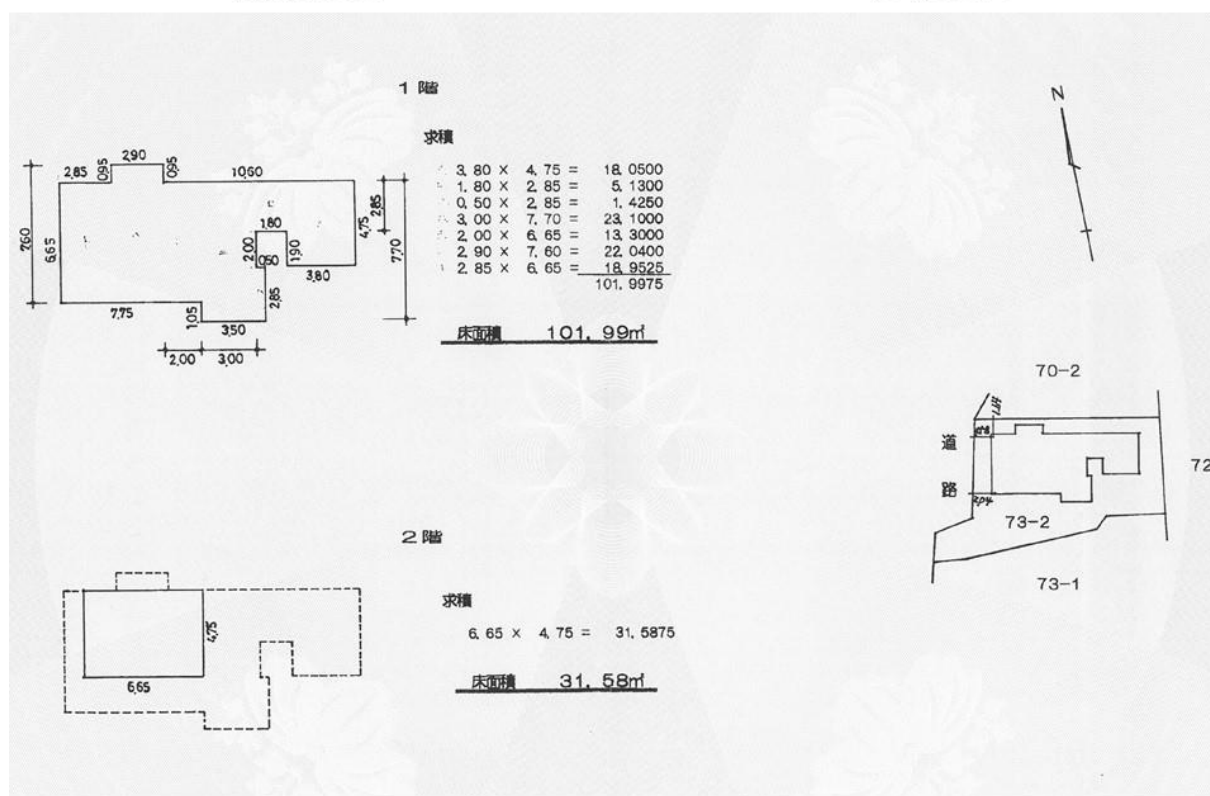
各階平面図
