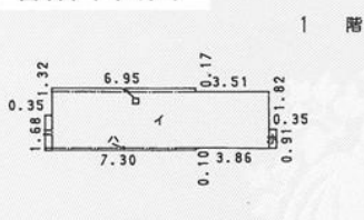
各階平面図
