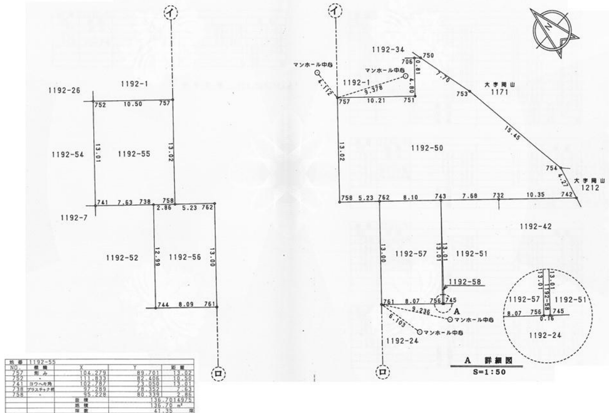
地積測量図
