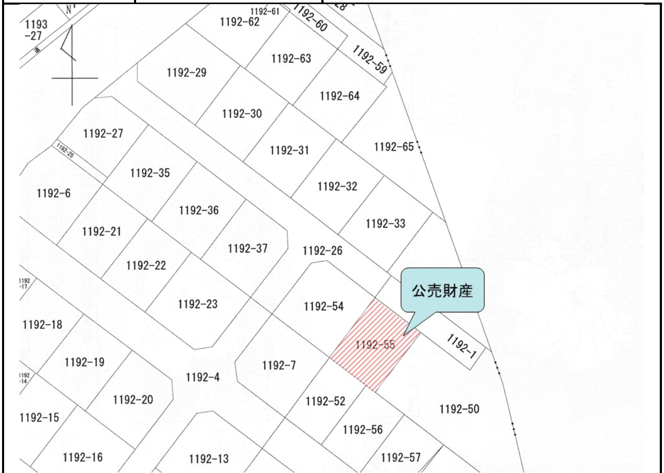
地積測量図
