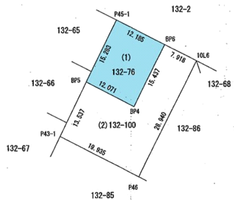
拡大図 1/500
