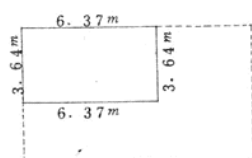
2階平面図
