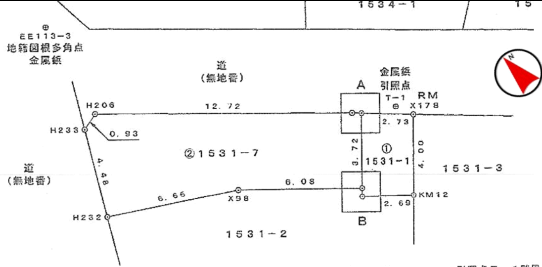
引照点 T-1 略図
