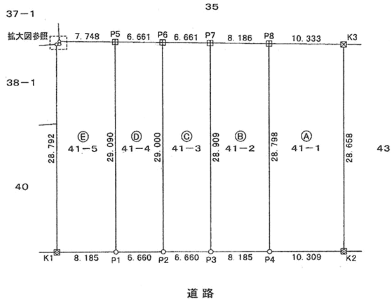
直角座標法求積表
